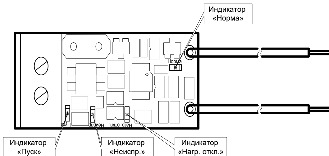
Рисунок 4 Расположение светодиодов
