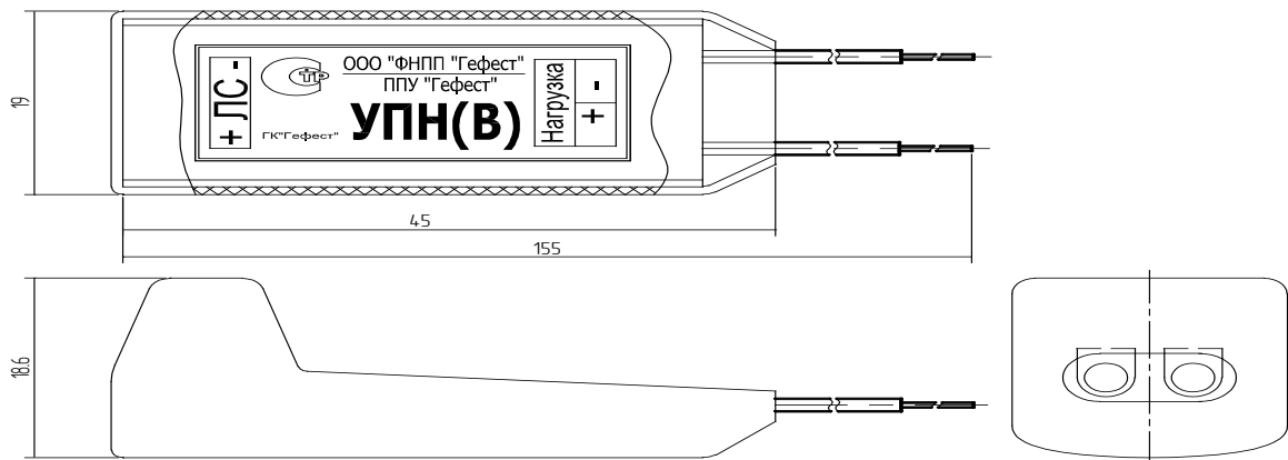
Рисунок 1 Внешний вид устройства (для УПН(С) надпись на корпусе соответственно «УПН(С)»)
