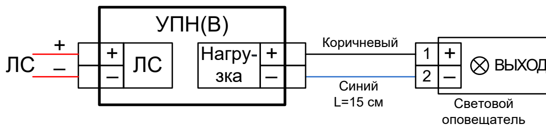
Рисунок 2 Схема подключения УПН(В)
