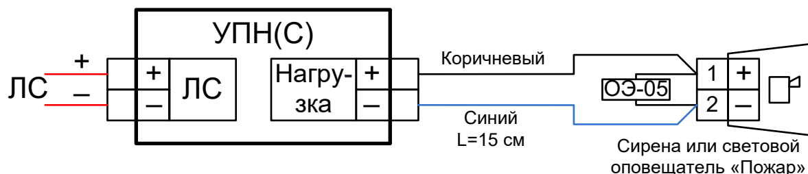
Рисунок 3 Схема подключения УПН(С)
